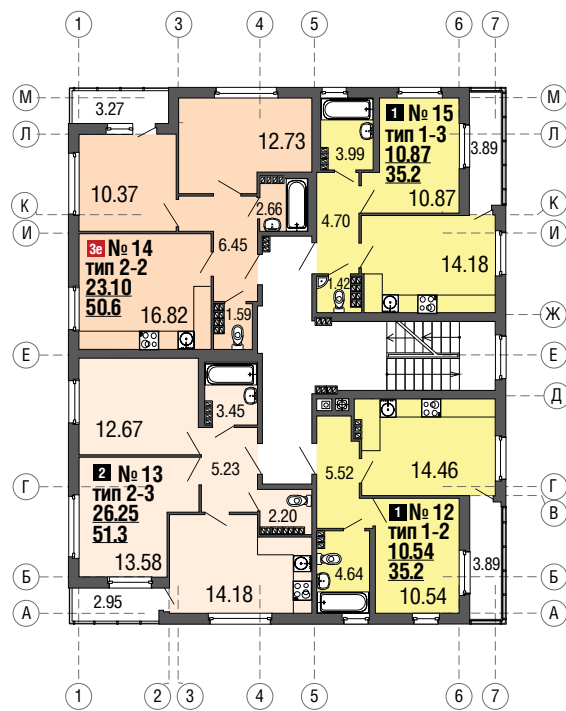
4 этаж
