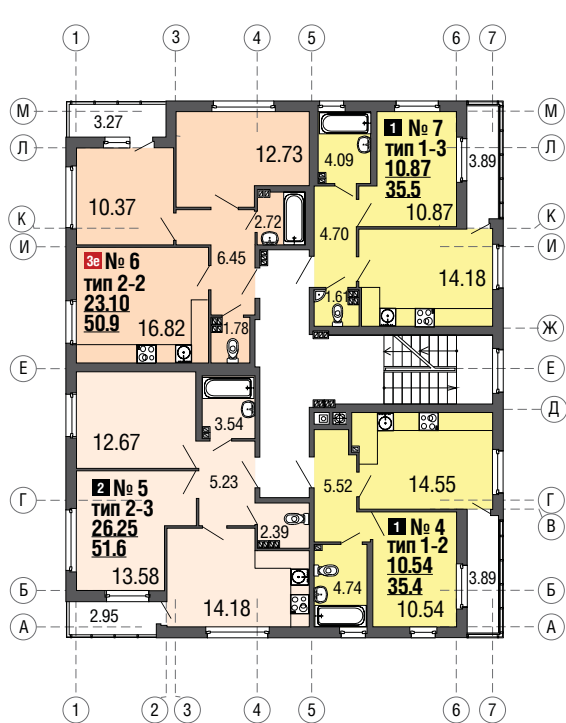
2 этаж
