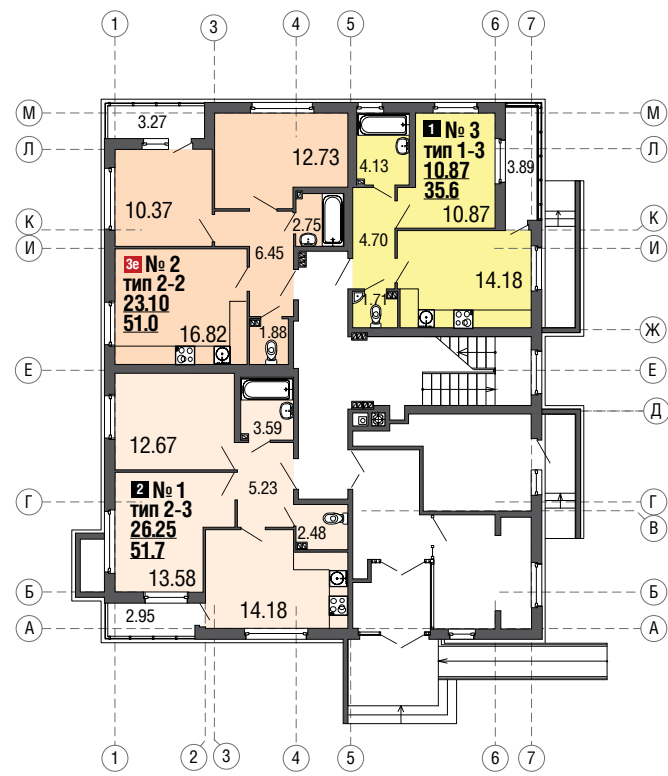
3 этаж
